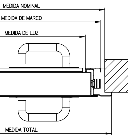
CORTE B-B
