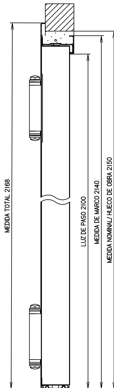
CORTE A-A 1:5
