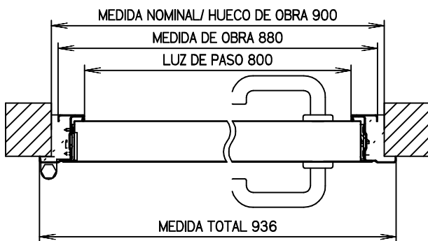
CORTE B-B 1:8
