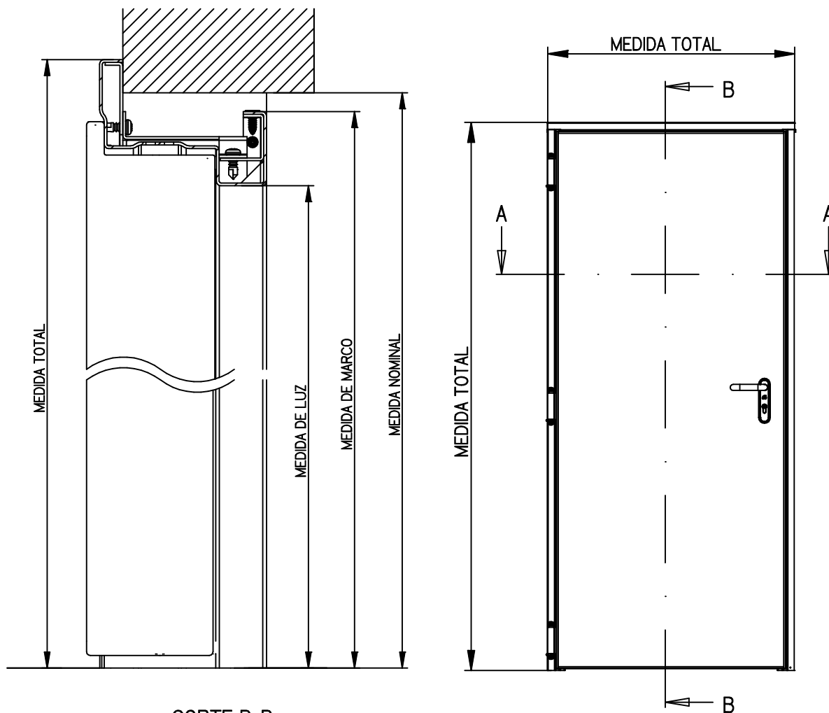
CORTE B-B 1:2.86
