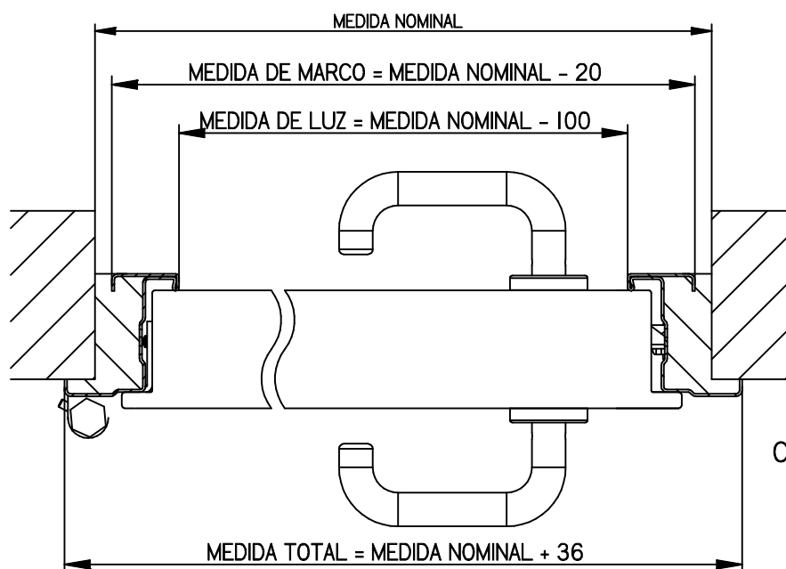
CORTE B-B 1:2.86
