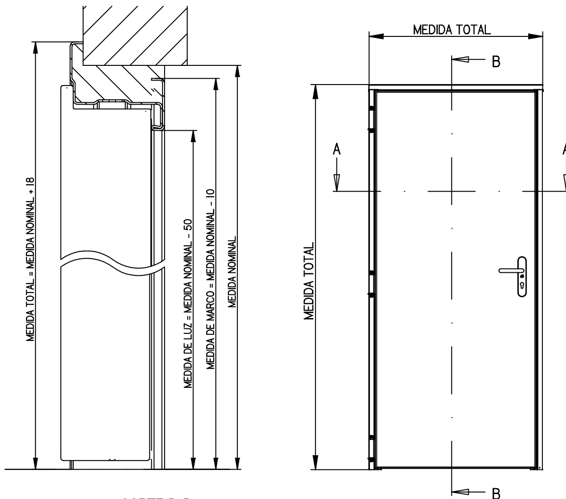
CORTE B-B 1:2.86
